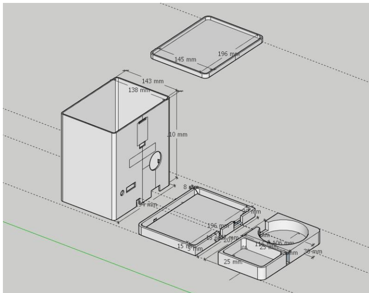
图 14 SketchUp 三维建模设计图视角 b
