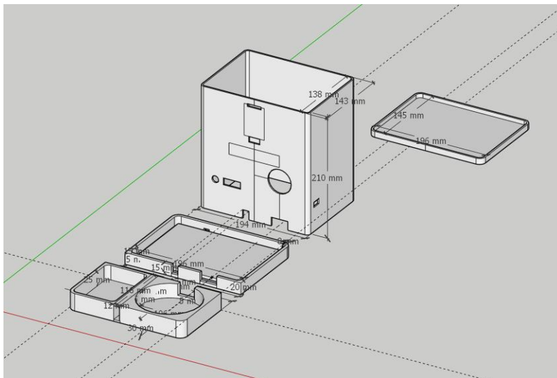
图 13 SketchUp 三维建模设计图视角 a
