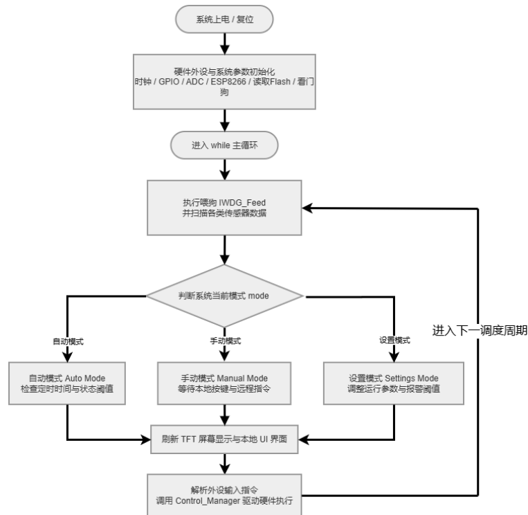
图 21 下位机主程序流程图
