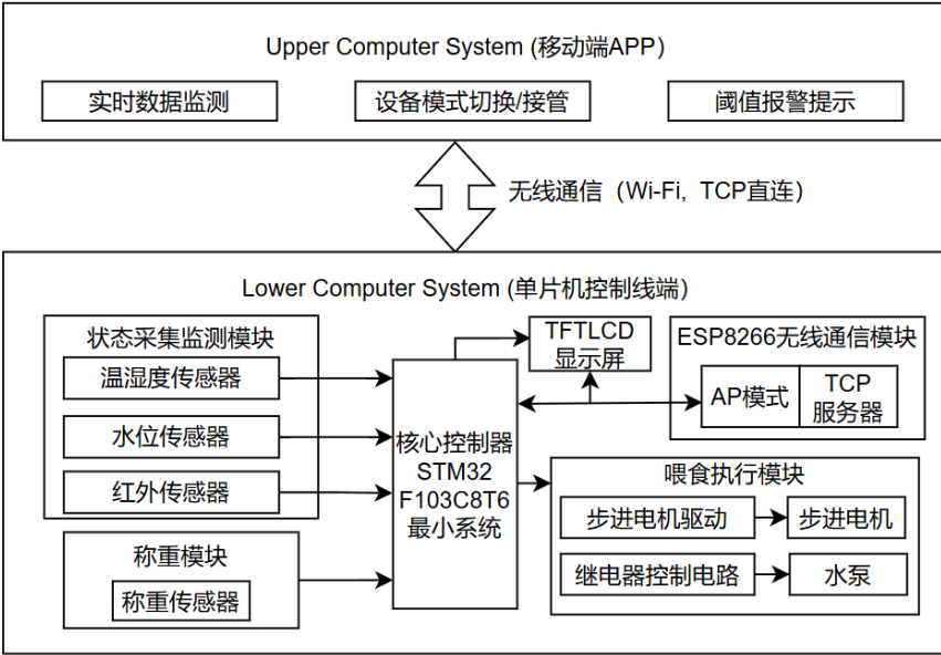
图 1 系统框图
