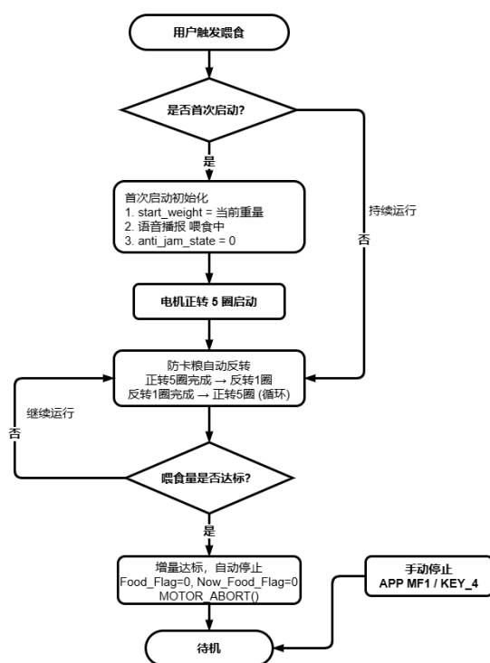
图 22 智能喂食流程图
