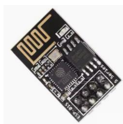
图 11 ESP8266Wi-Fi 模块
