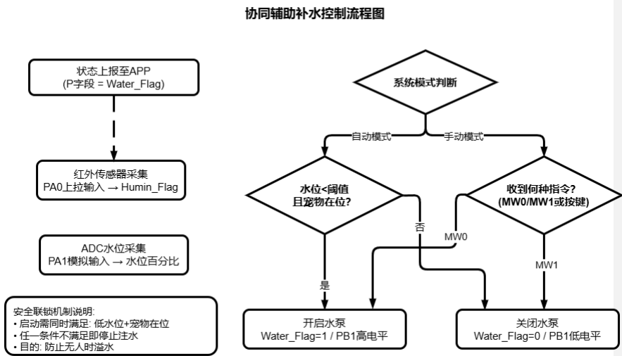
图 23 协同辅助补水流程
