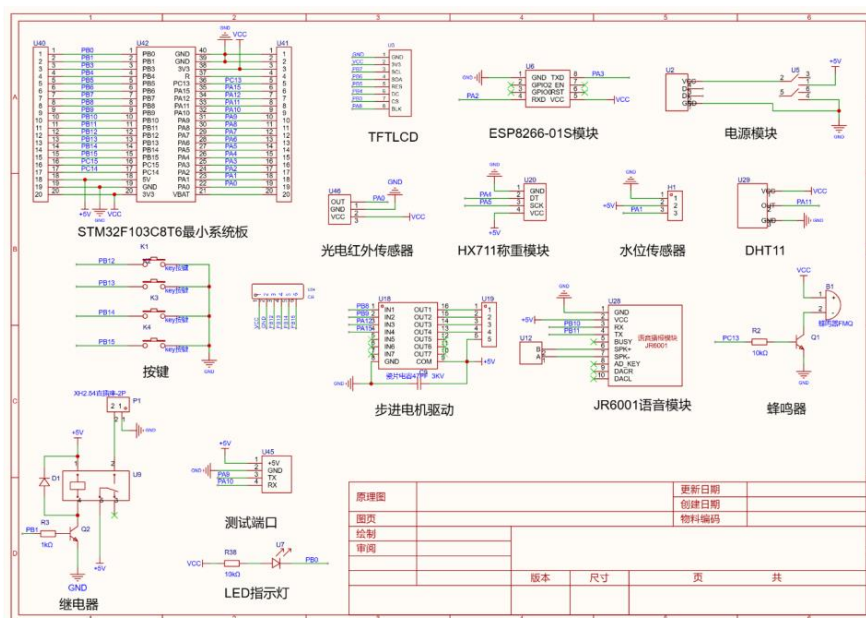
图 15 原理图
